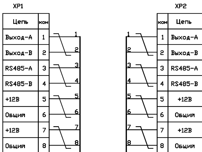
Рис.2. Кабель связи.
