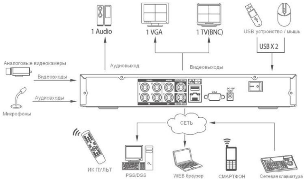
Рис. 2.3-1 Видеорегистратор RVi-04LA
