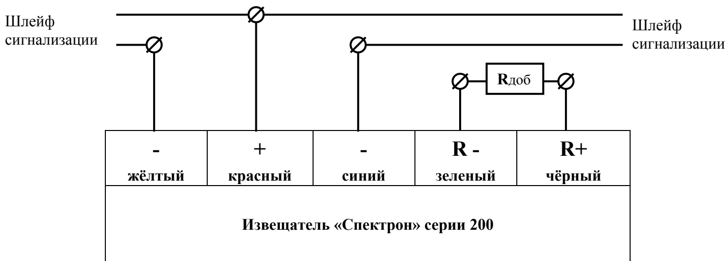
Рис. 8 Схема включения извещателя
