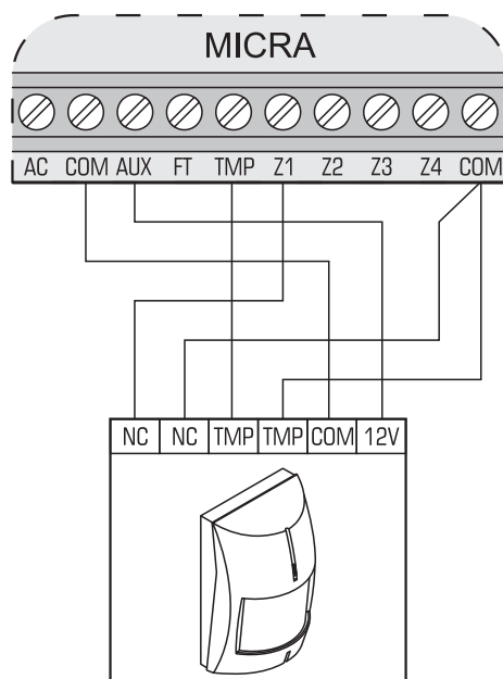
Рис. 5. Пример подключения извещателя типа NC к модулю MICRA (извещатель типа NO подключается аналогично).
