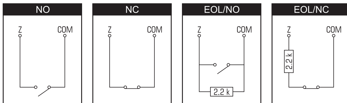
Рис. 4. Способы подключения извещателей к охранному модулю.
