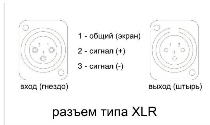
Рис.1 Функциональное назначение контактов разъемов линейных входа и выхода
