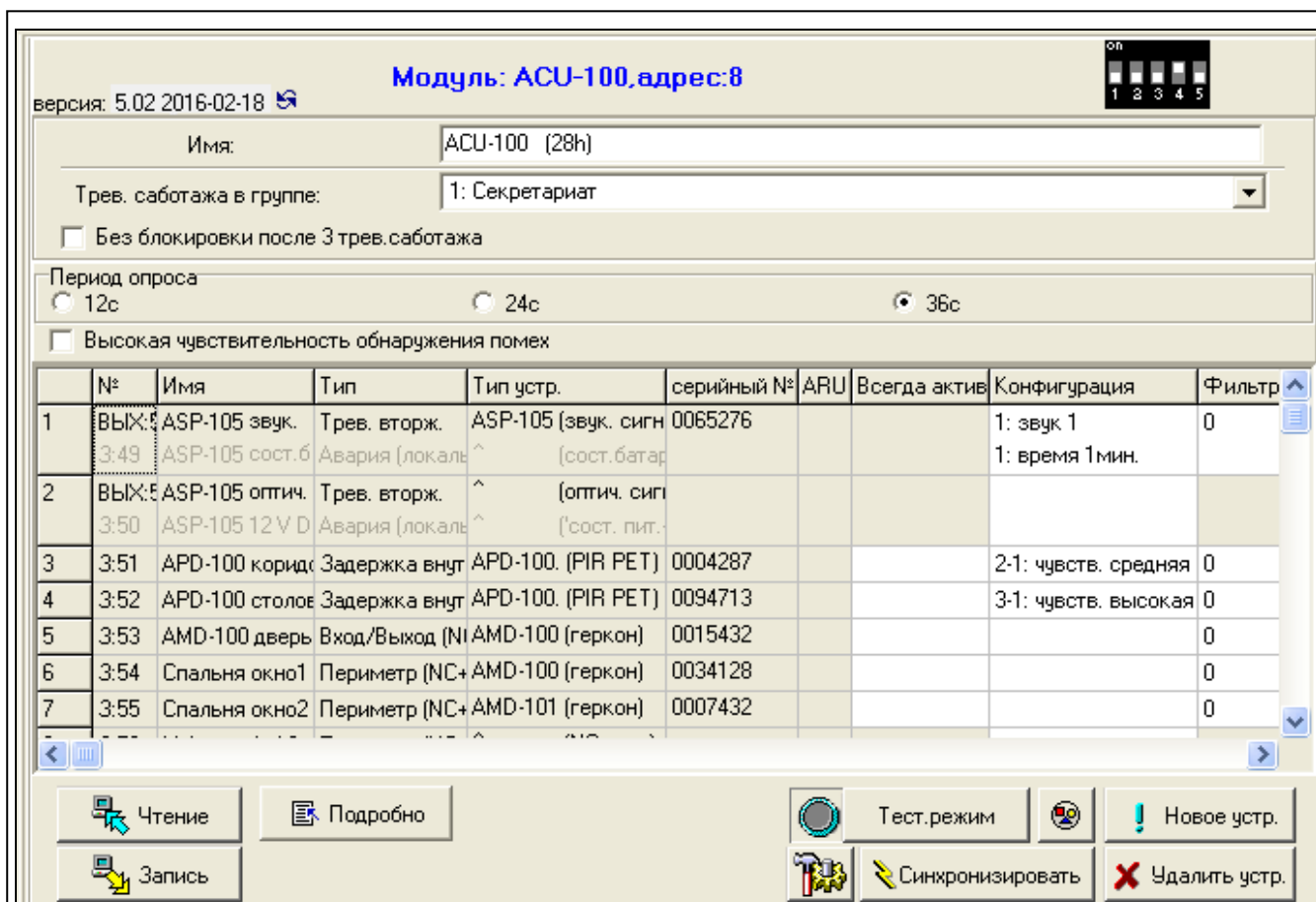
Рис. 4. Программа DLOADX: список беспроводных устройств, зарегистрированных в контроллере, подключенным к прибору INTEGRA / INTEGRA Plus.
