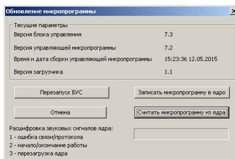
Рисунок 7.53. Диалоговое окно обновления микропрограммы главного микроконтроллера БУС.
