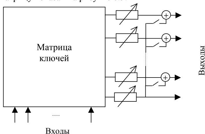
Рисунок 6.5. Схема прохождения сигнала через аналоговую матрицу.
