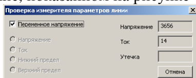
Рисунок 7.56. Диалоговое окно проверки измерителя импеданса.
