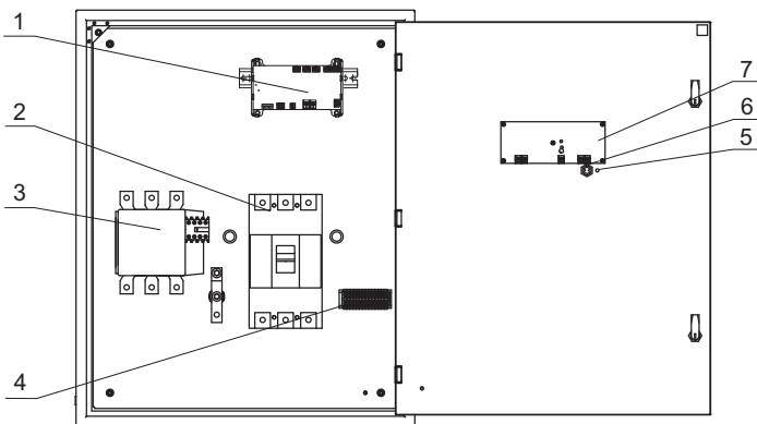
в) ШУ мощностью 55-110 кВт
