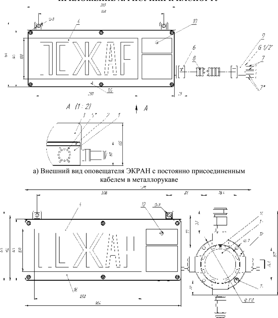
б) Внешний вид оповещателя ЭКРАН-ККВ с постоянно присоединенной внешней взрывозащищенной клеммной коробкой
