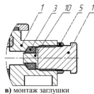
в) монтаж заглушки
