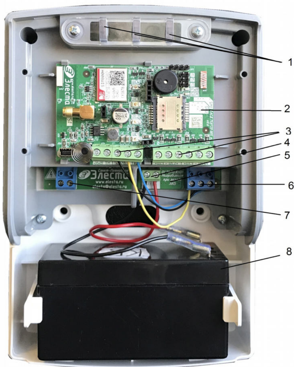
Рисунок 2.5 - Прибор Юпитер-2428 с открытой крышкой
