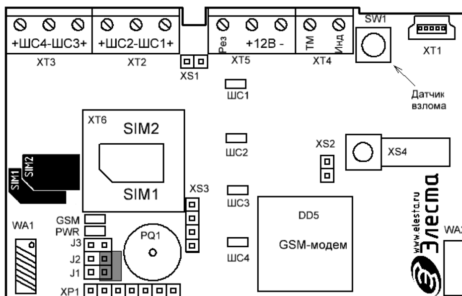
Рисунок 3.3 - Плата версии 0.6 и 0.7. Взаимное замыкание переключек
