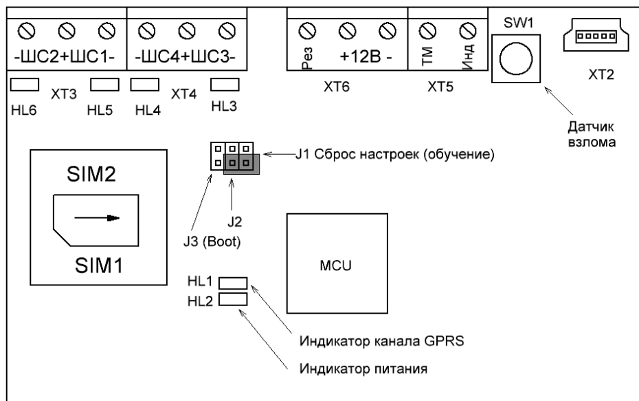
Рисунок 3.2 - Плата версии 0.2. Взаимное замыкание переключек
