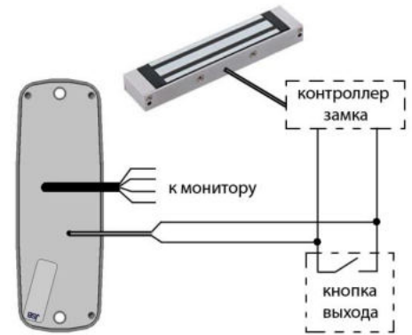
Схема подключения электромагнитного замка
