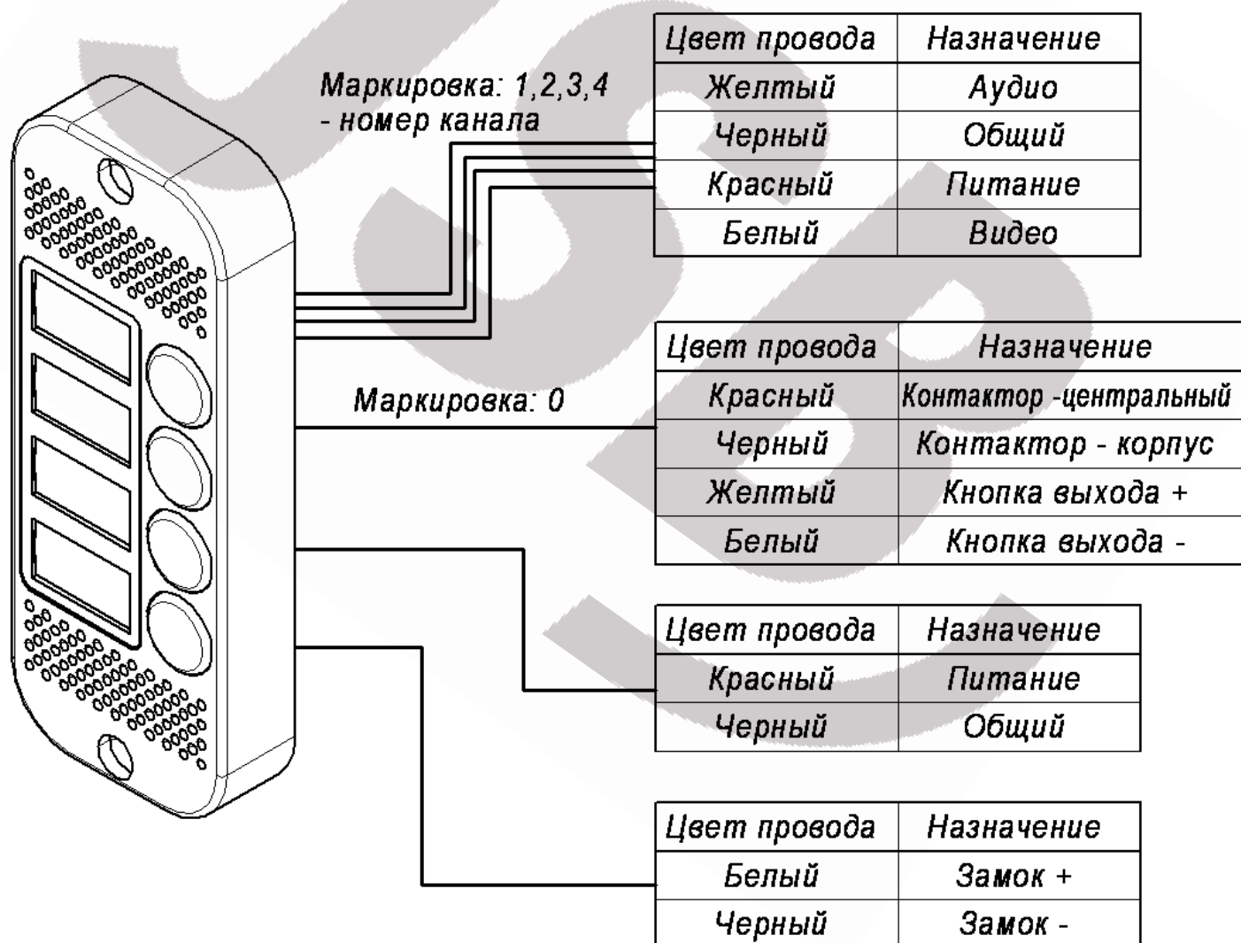
Рис.2 Схема подключения панели.
