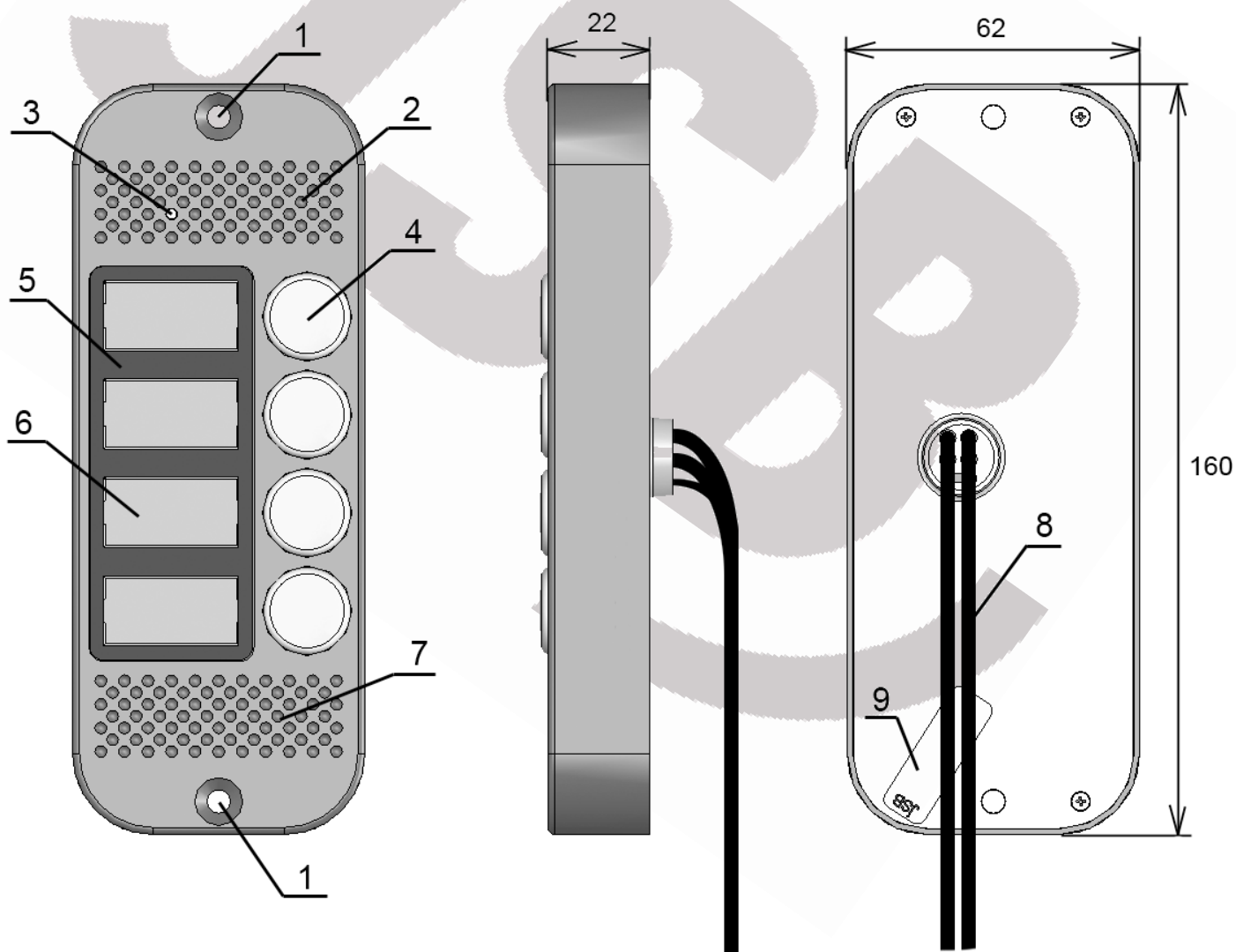
Рис. 1. Назначение основных узлов панели:
