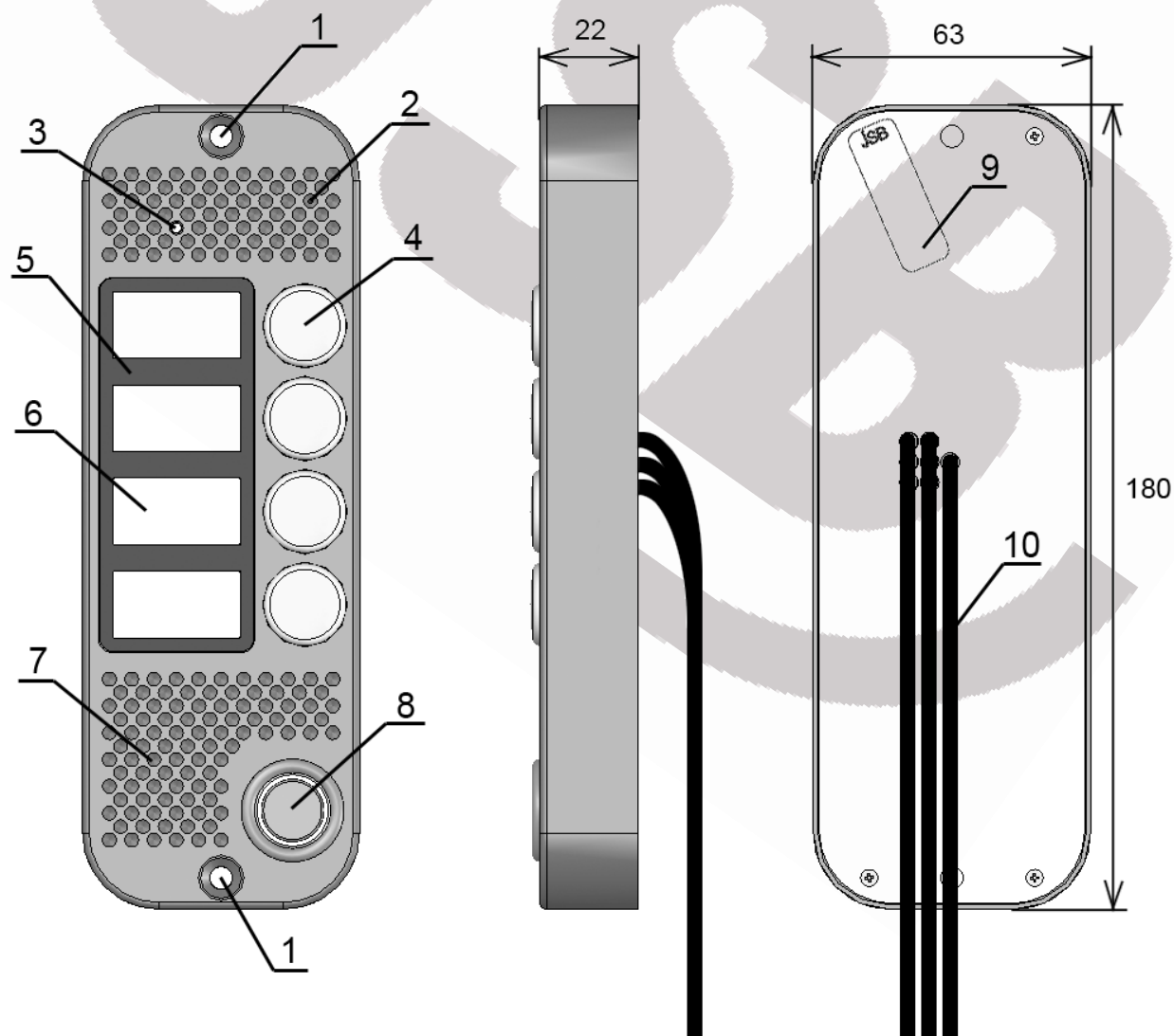
Рис. 1. Назначение основных узлов панели:
