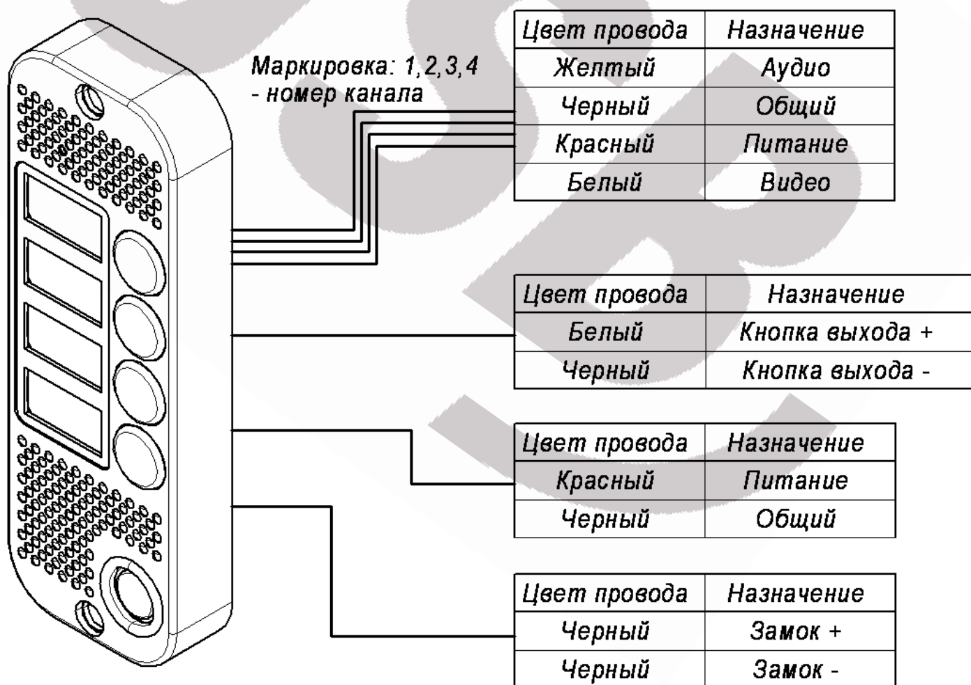
Рис.2 Схема подключения панели.
