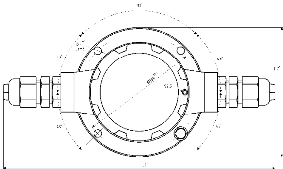
Рисунок 2. Габаритные и установочные размеры коробки ККВ-07е-II.
