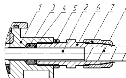
а) монтаж бронированным кабелем или металлорукавом
