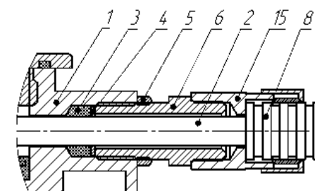
б) монтаж кабелем в металлорукаве
