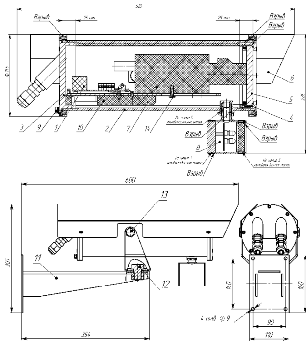
1 – плата клемм; 2 – корпус; 3 – задняя крышка; 4 – передняя крышка; 5 – стекло; 6 – козырек (опция); 7 – видеокамера с объективом (опция); 8 – инфракрасная подсветка (опция); 9 – винт М6 заземления; 10 – направляющая; 11 – кронштейн; 12, 13 – болты крепления термокожуха к кронштейну; 14 – винт 1/4" крепления видеокамеры.
