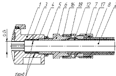
е) монтаж бронированным кабелем в кабельном вводе КВБУ
