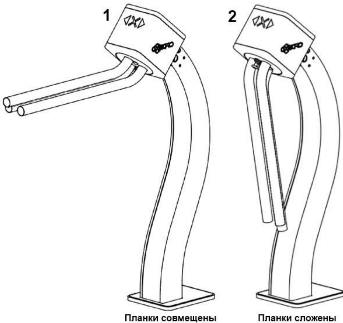
Рисунок 7 – Положения планок
