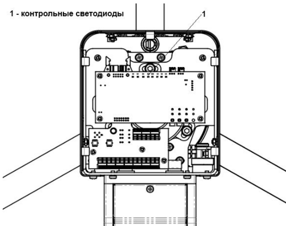
Рисунок 11 – Расположение контрольных светодиодов на материнской плате
