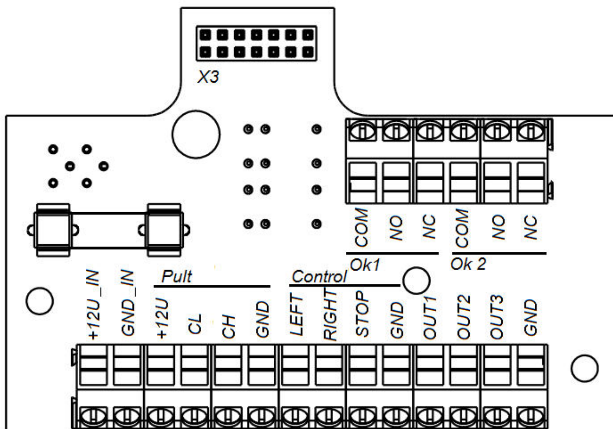
Рисунок 9 – Внешний вид кросс-платы
