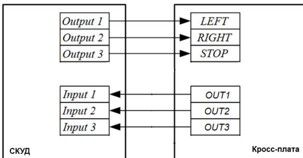
Рисунок 14 – Схема подключения ПУ к контроллеру СКУД
