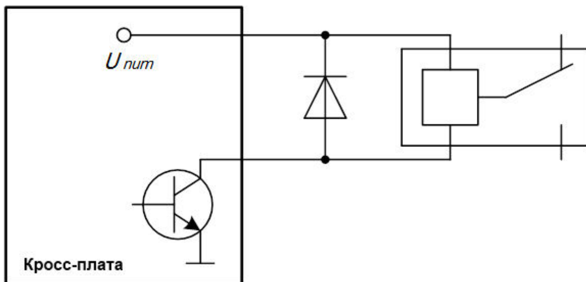
Рисунок 13 – Схема подключения диода параллельно обмотке реле
