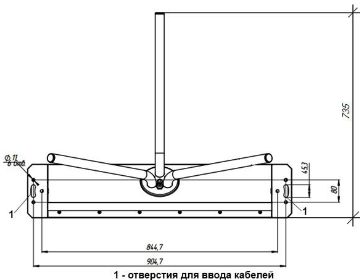
Рисунок 6 – Установочные размеры турникета
