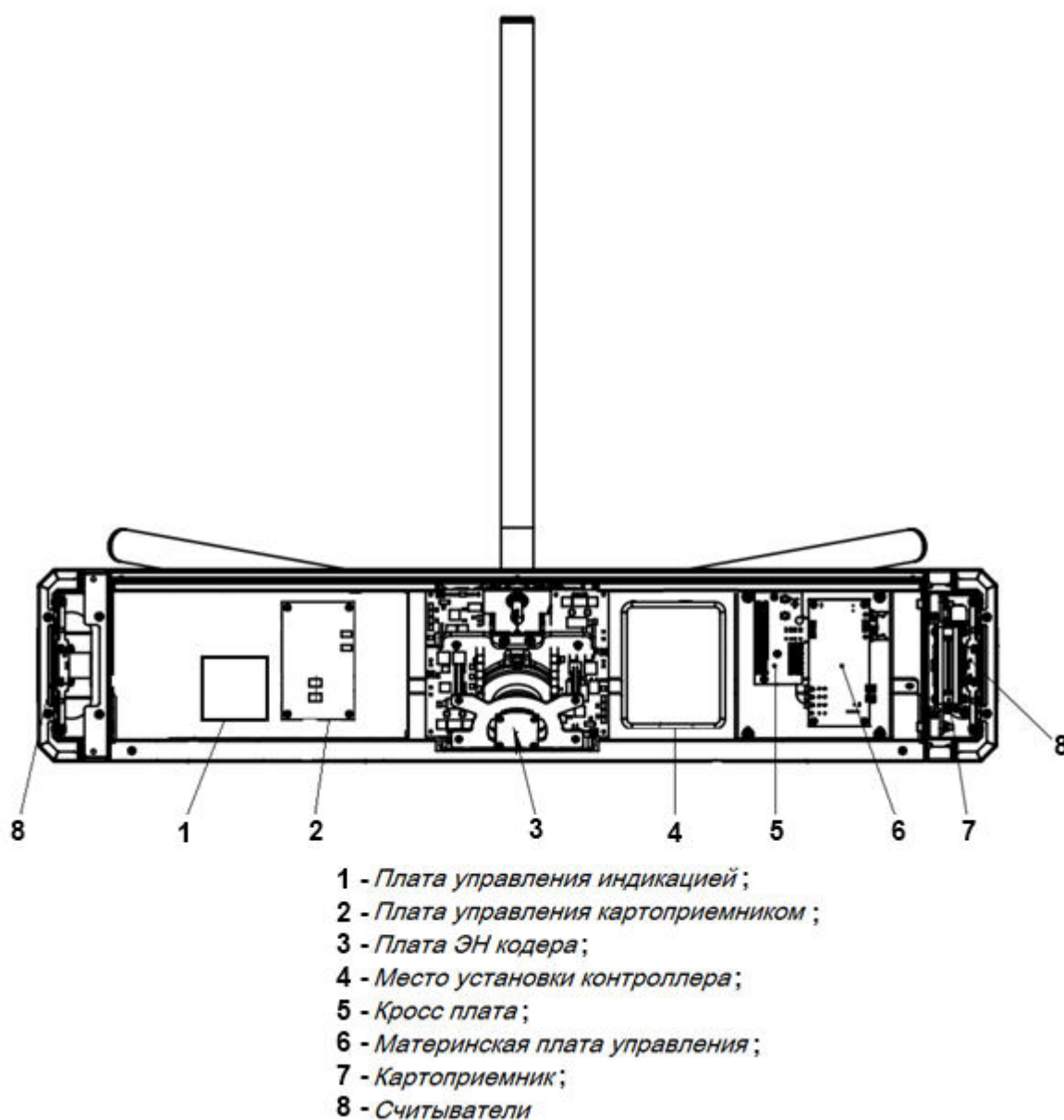
Рисунок 8 – Расположение плат под верхней крышкой
