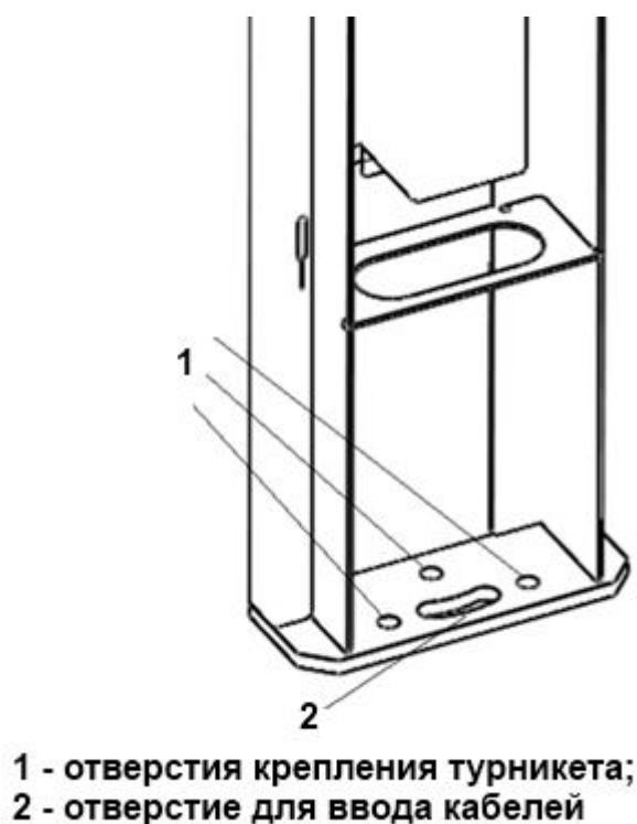
Рисунок 5 – Стойка турникета
