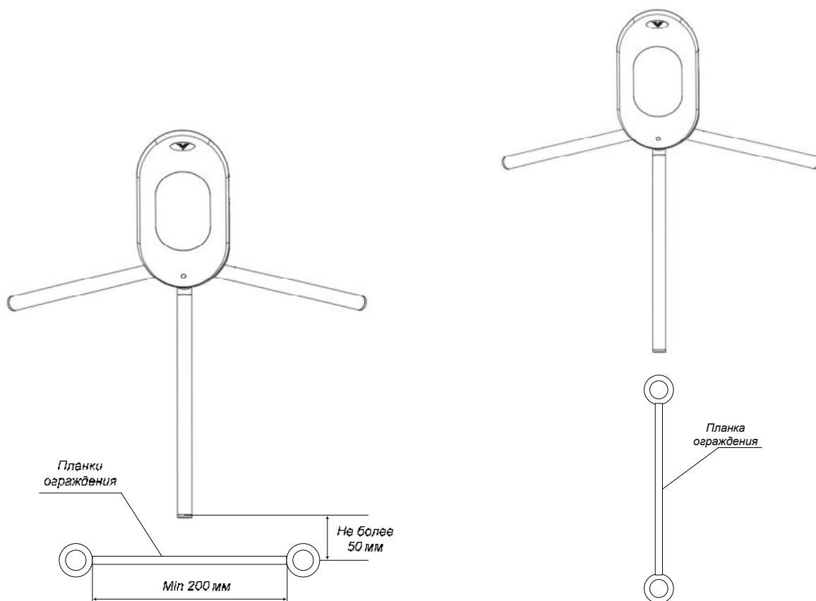
Рекомендованная схема установки
