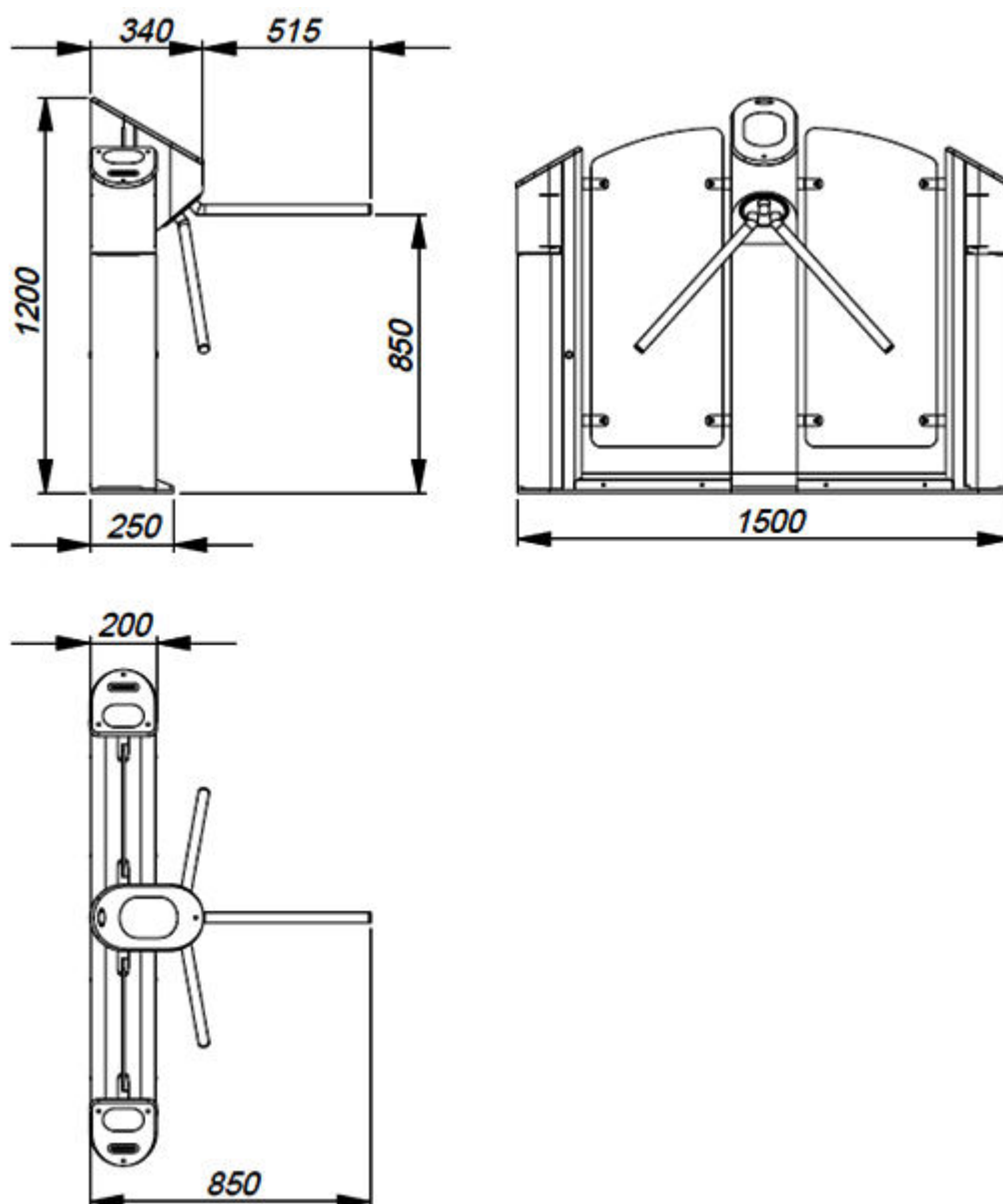
Рисунок 1 – Габаритные размеры турникета
