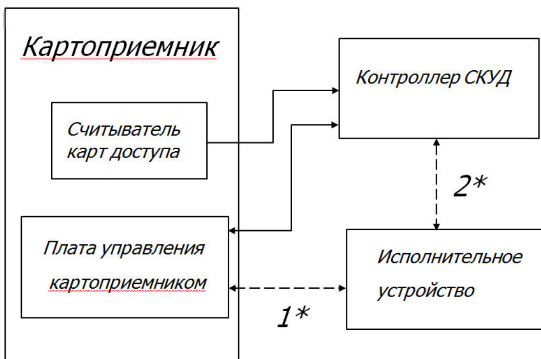
Рисунок 19 – Структурная схема №3
