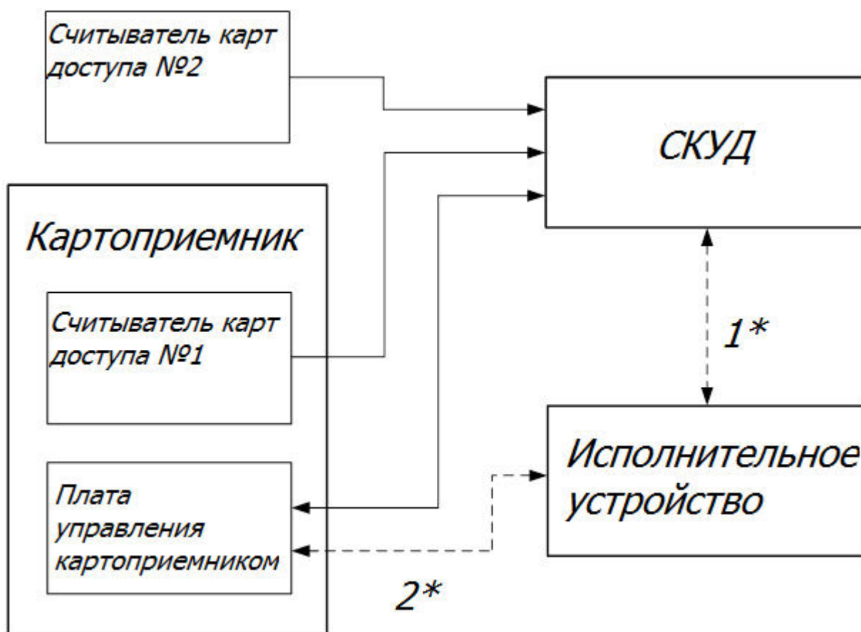
Рисунок 16 – Структурная схема №1
