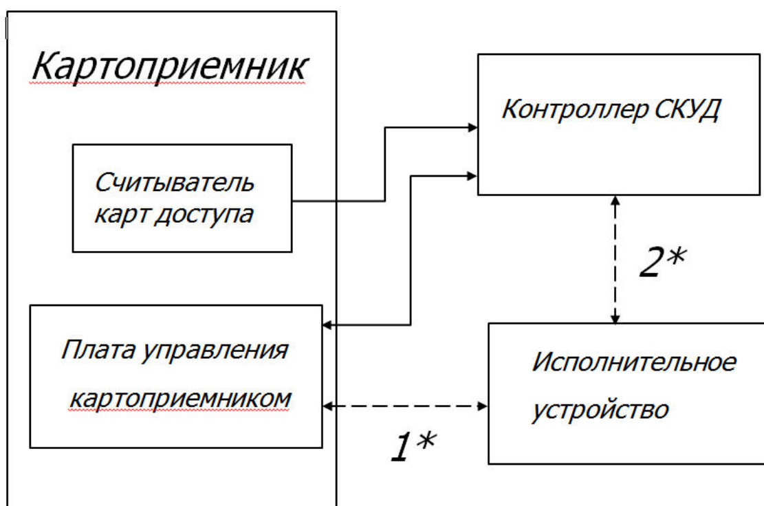
Рисунок 18 – Структурная схема №3
