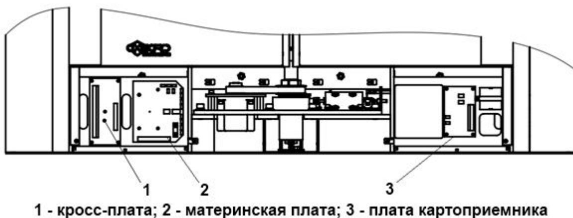
Рисунок 4 – Расположение плат на стойке модуля турникета
