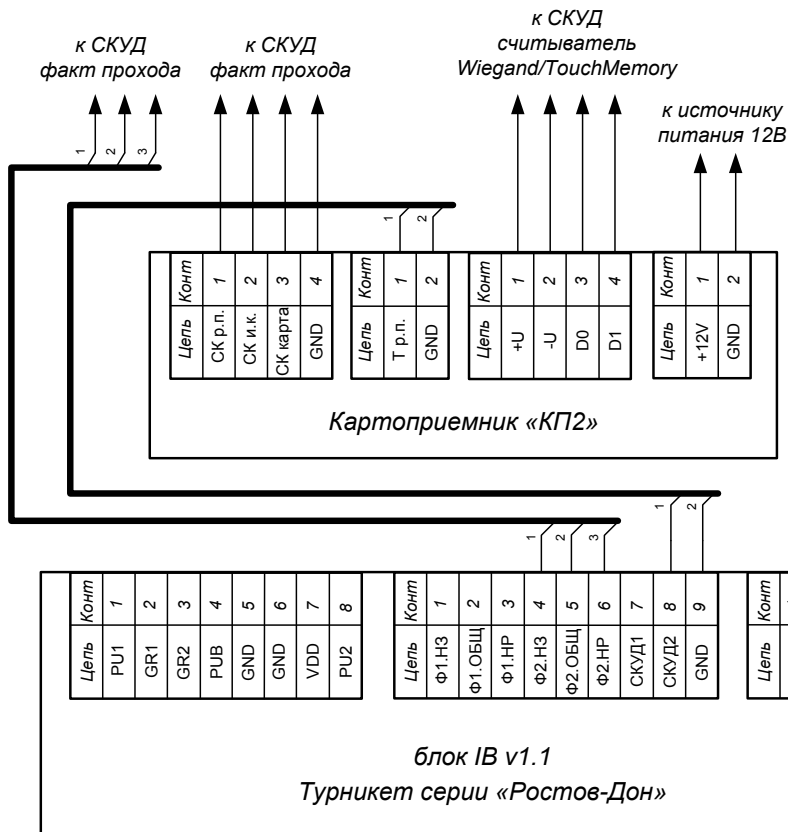
Схема электрическая подключения картоприемника «Ростов-Дон КПМ» к турникету серии «Ростов-Дон»
