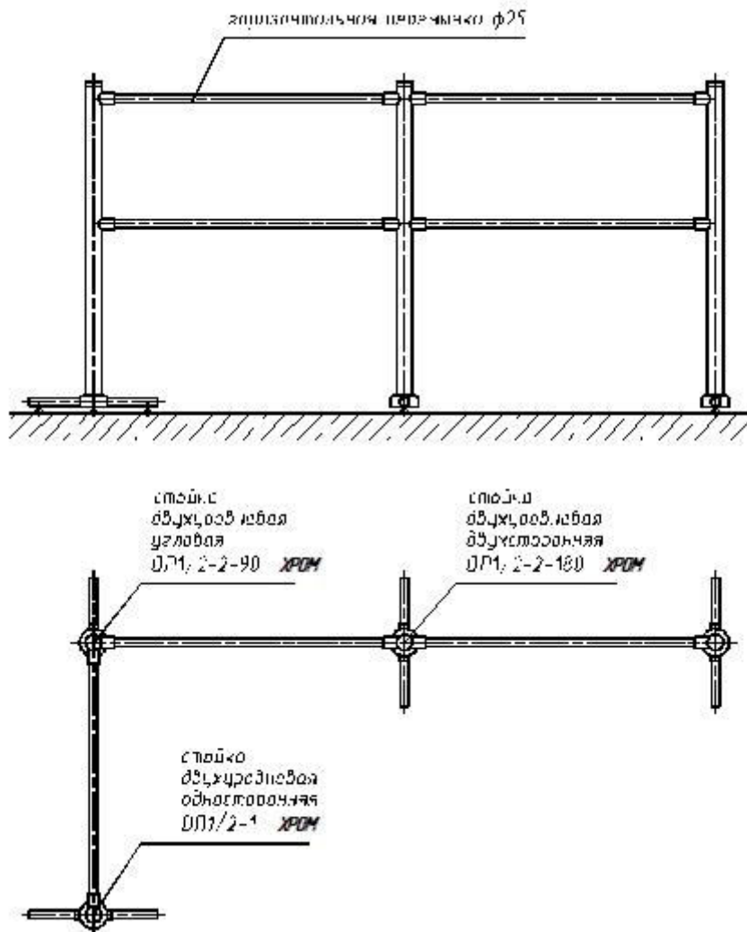
Пример компоновки ограждений ОП1
