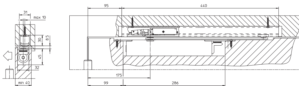
Fig. 06-1 · GEZE Boxer – сила закрывания 2-4 со скользящей шиной E для доводчика Boxer
