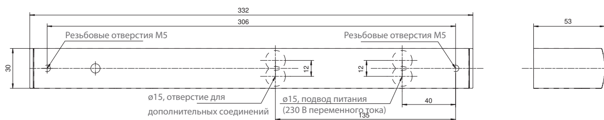
Fig. 15-1 · Габаритные размеры центрального пульта сигнализации о задымлении RSZ6
