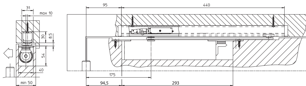
Fig. 06-2 · GEZE Boxer – сила закрывания 3-6 со скользящей шиной E для доводчика Boxer
