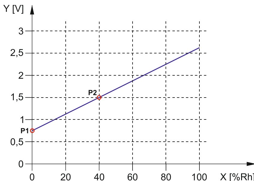
Рис. 22. Пример линейной характеристики датчика влажности воздуха.
