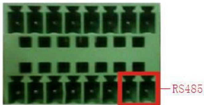
485 порт восьмиканального наружного устройства
