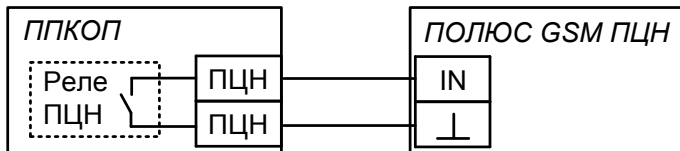
Рис.7 Схема подключения к ППКОП
