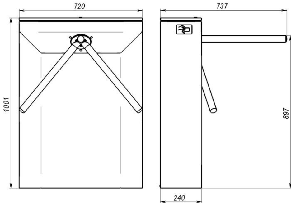
Рис.6 Турникет. Габаритные размеры
