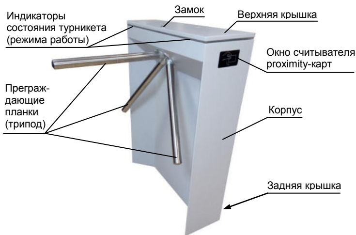
Рис.1 Общий вид турникета
