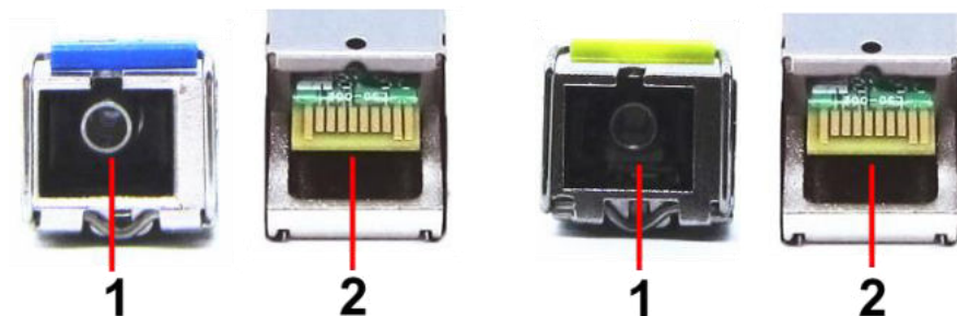
Рис. 3 SFP модули SFP-S1SC19-G-1310-1550, SFP-S1SC19-G-1550-1310, разъемы
