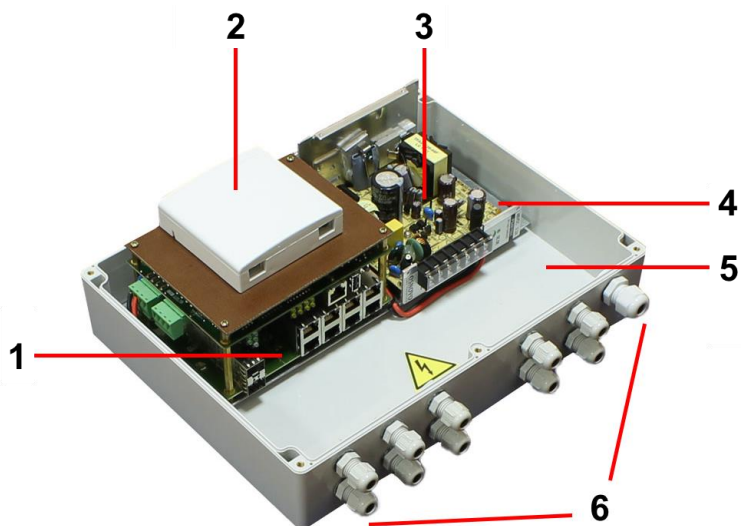
Рис.2 Уличный коммутатор SW-80802/WLC, основные элементы
