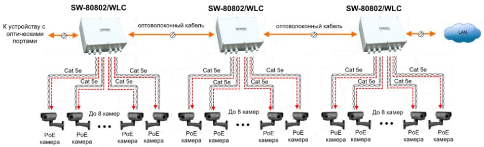
Рис.5 Каскадная схема подключения коммутатора SW-80802/WLC,
