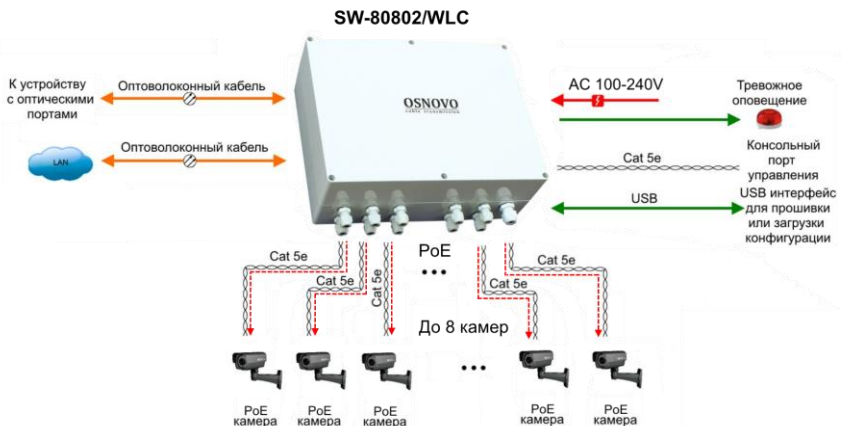
Рис.6 Типовая схема подключения коммутатора SW-80802/WLC
