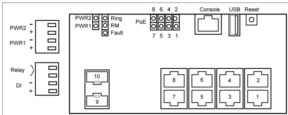
Рис. 3 Уличный коммутатор SW-80802/WLC, разъемы кнопки и индикаторы
