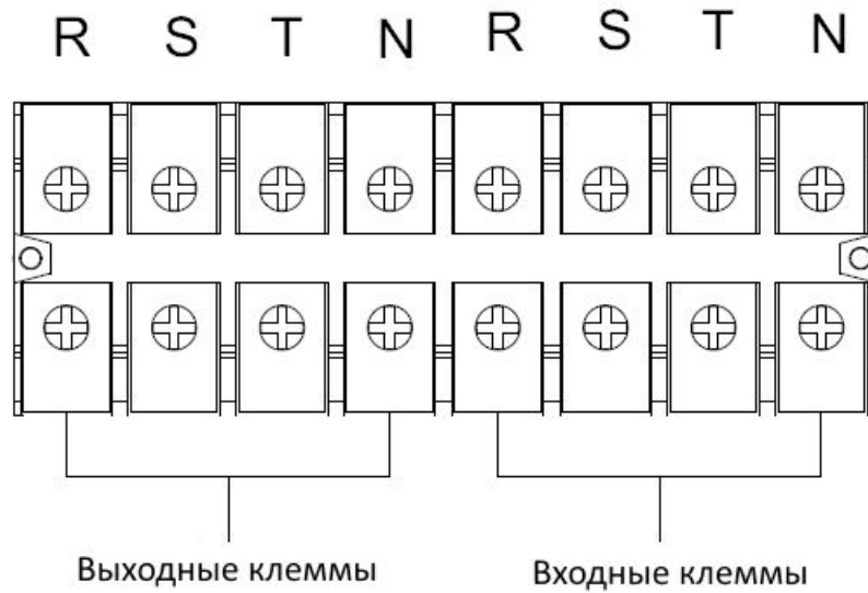
Рис. 2-3-1 Блок клемм ИБП XE 30(WB) / 40(WB)
