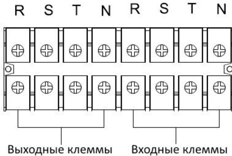
Рис.2-3-2 Блок клемм ИБП XE 60 / 80
