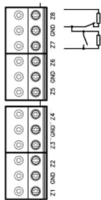
Рис.15. Подключение шлейфов блокировки и свободного прохода
