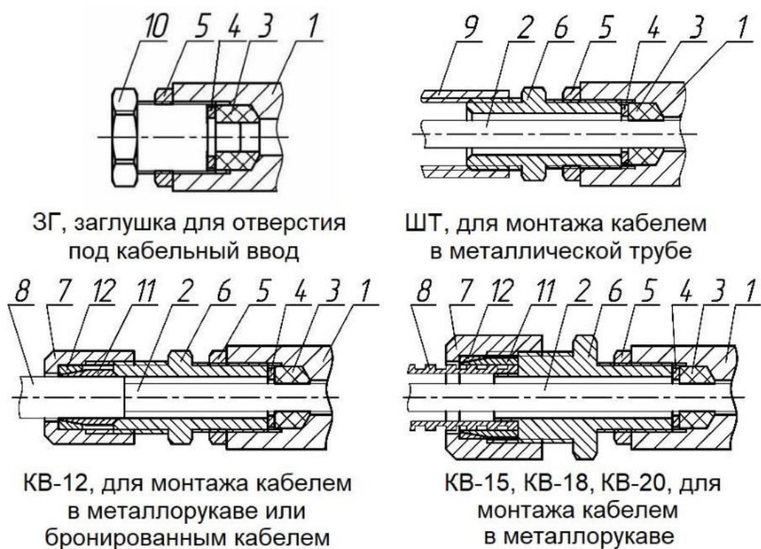
Рисунок 12 – Вводные устройства с одинарным уплотнением
