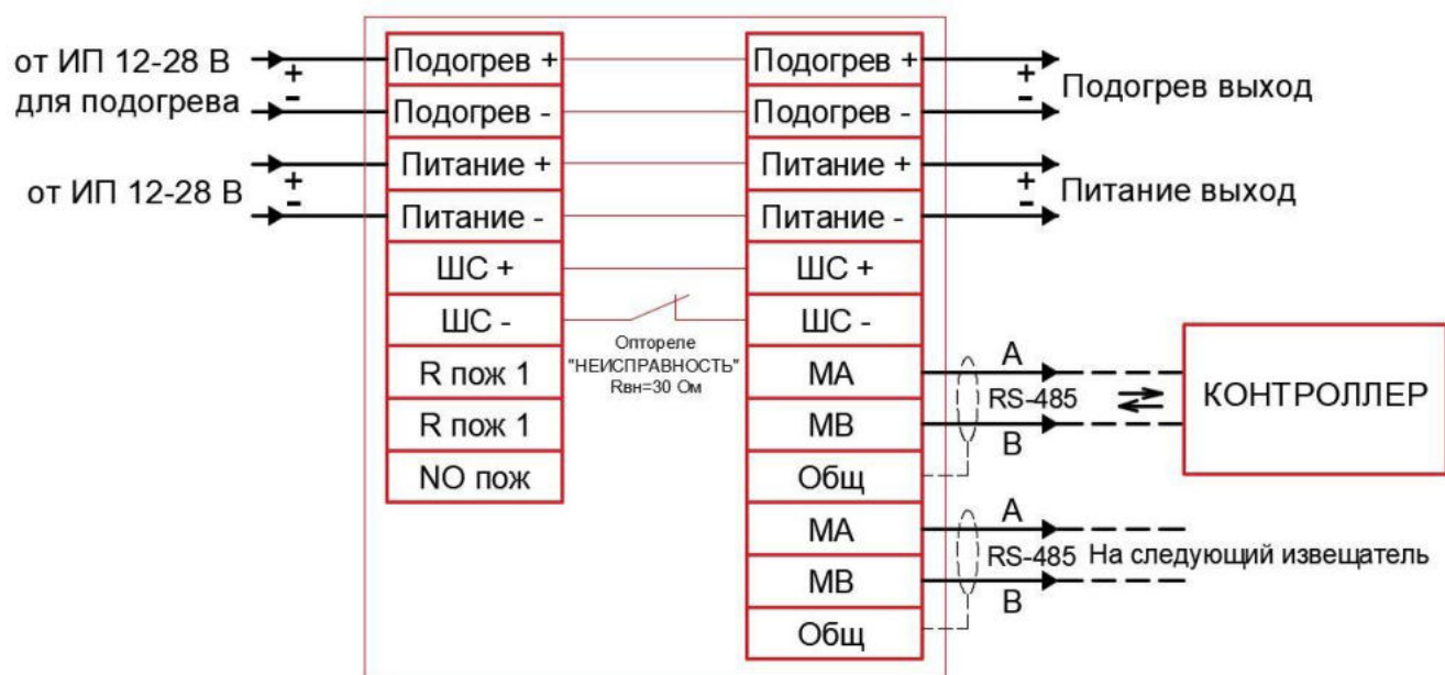
Рисунок 9 – Схема подключения по интерфейсу RS-485
