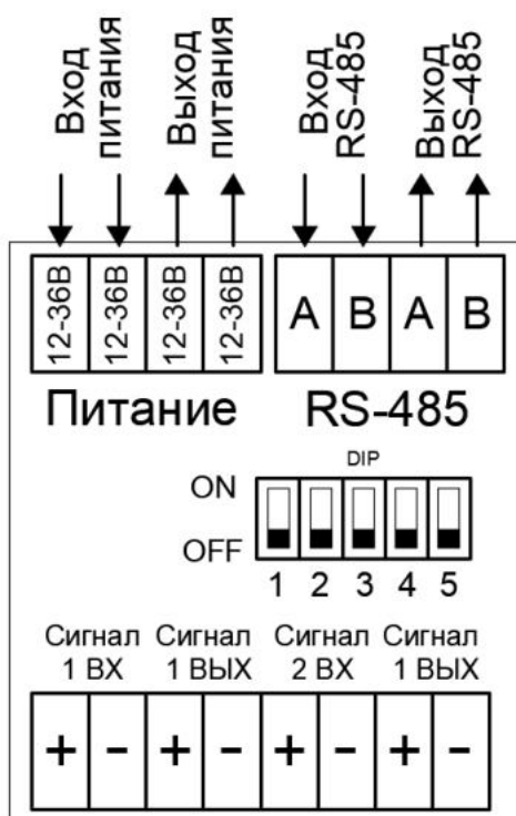
Рис. 3 Схема двухпроводного подключения оповещателя 12-36 В DC
