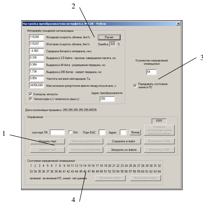
Рисунок 7.1. Окно ПО. 1 – Основные органы управления, 2 – настройки интерфейса с ПС, 3 – настройка режима работы БСПС, 4 – состояния НПО.
