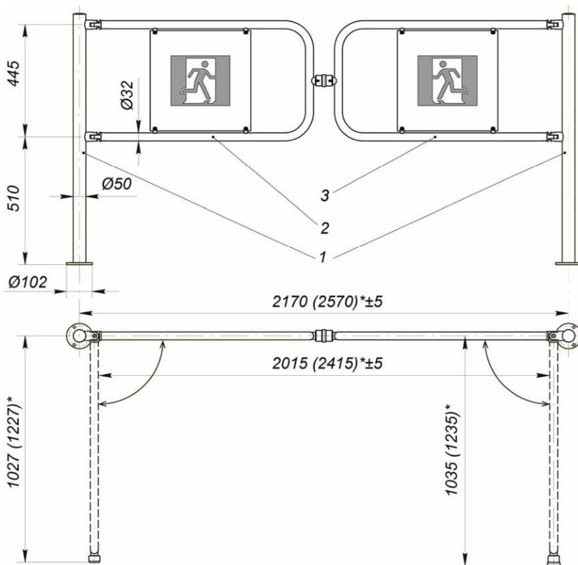
Рисунок 7. Двойная распашная секция ограждения с магнитным УБ 1 : 1 – стойка ВН02 2-00(01,02,03); 2 – створка ВН02 1-18(19) с магнитным УБ; 3 – створка ВН02 1-18(19) с ответной частью магнитного УБ
