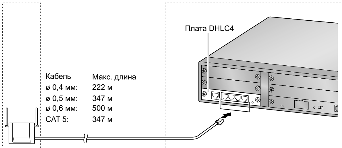
Плата DHLC/DLC (RJ45)
